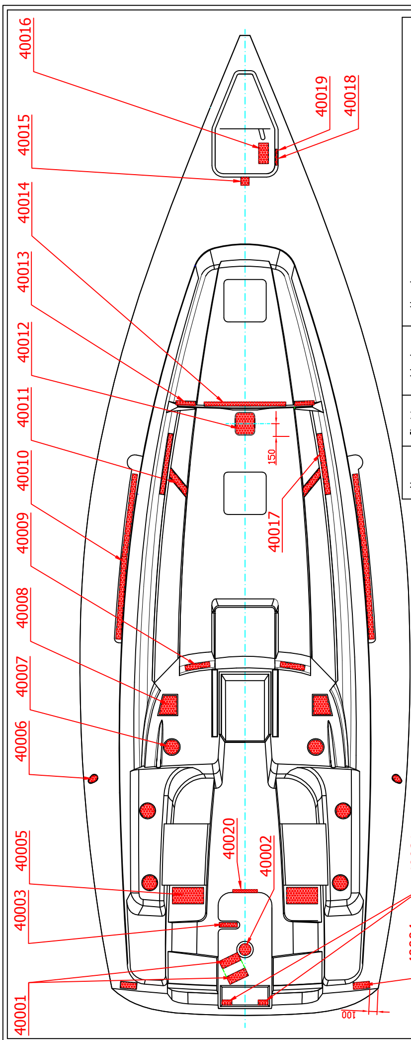
WYKAZ WZMOCNIEŃ METALOWYCH. List of metal reinforcements.
