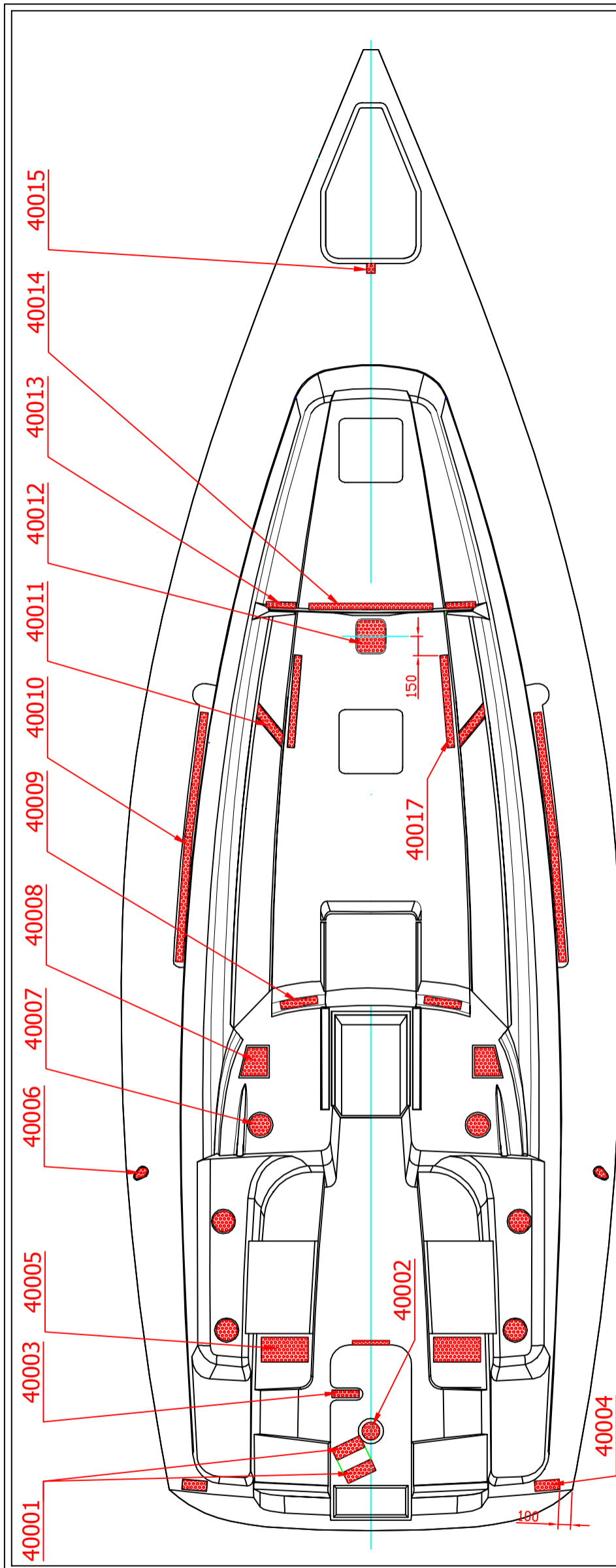
WYKAZ WZMOCNIENI METALOWYCH. List of metal reinforcements.
